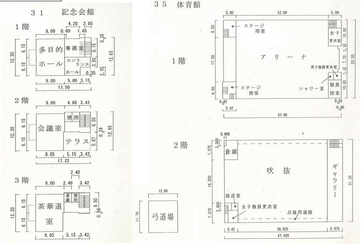
施設平面図
