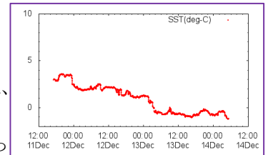
海水温
